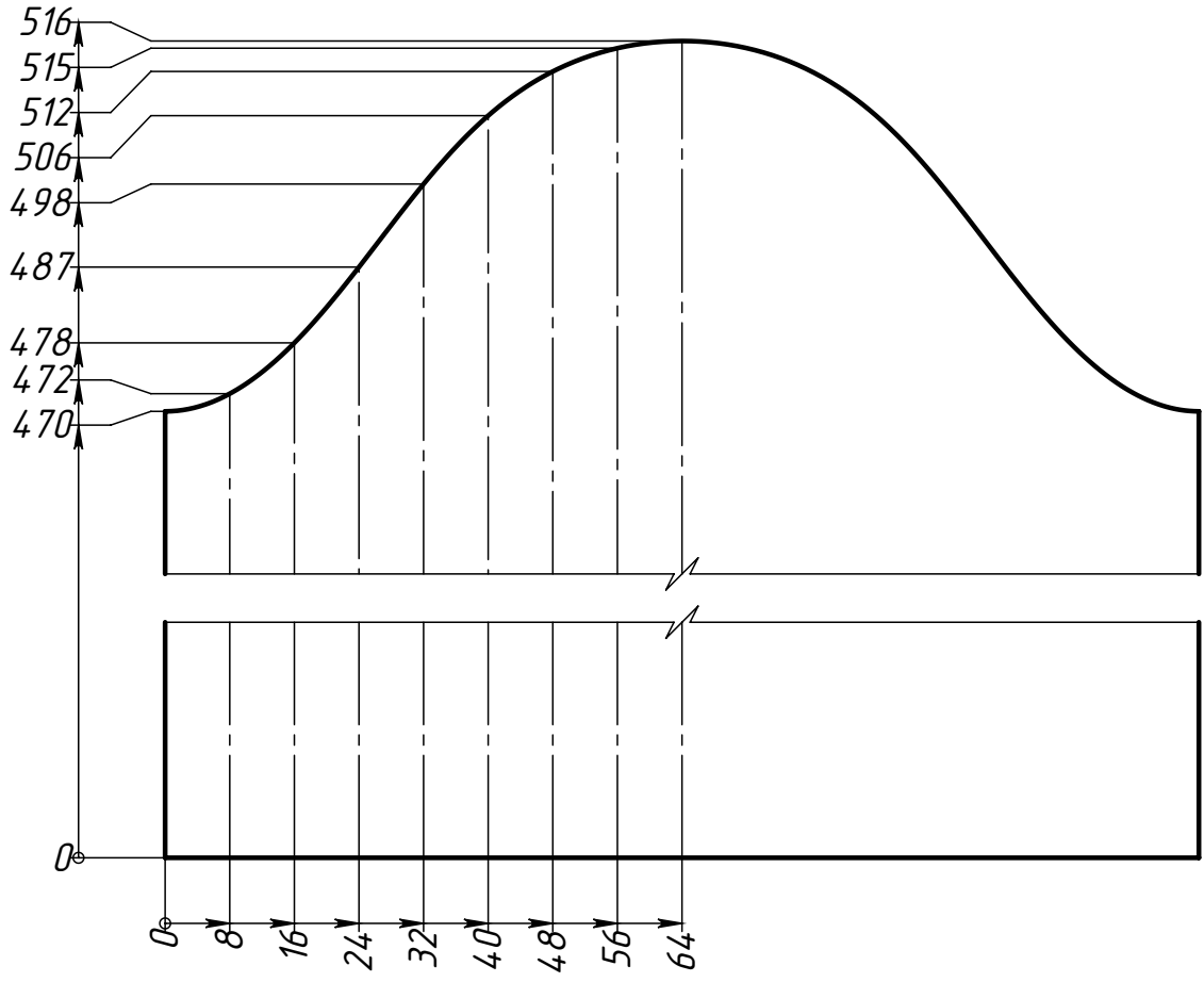
Поз.4 (Труба) Развертка 1 : 1
